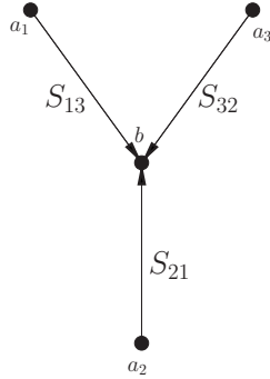
FIG. 17. The digraph T' .
